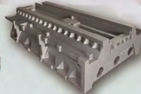
机床床身系列铸件
